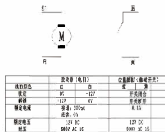
控制接线 Control Wiring
