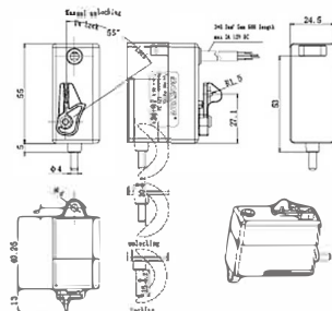
外形尺寸 Appearance dimensions
